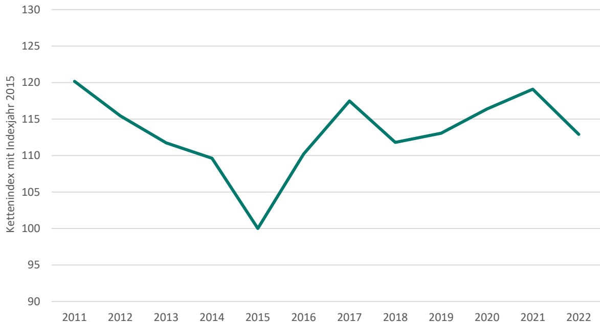
Abbildung 4-3 Entwicklung der energetischen realen Investitionen im Wohnungsbau
